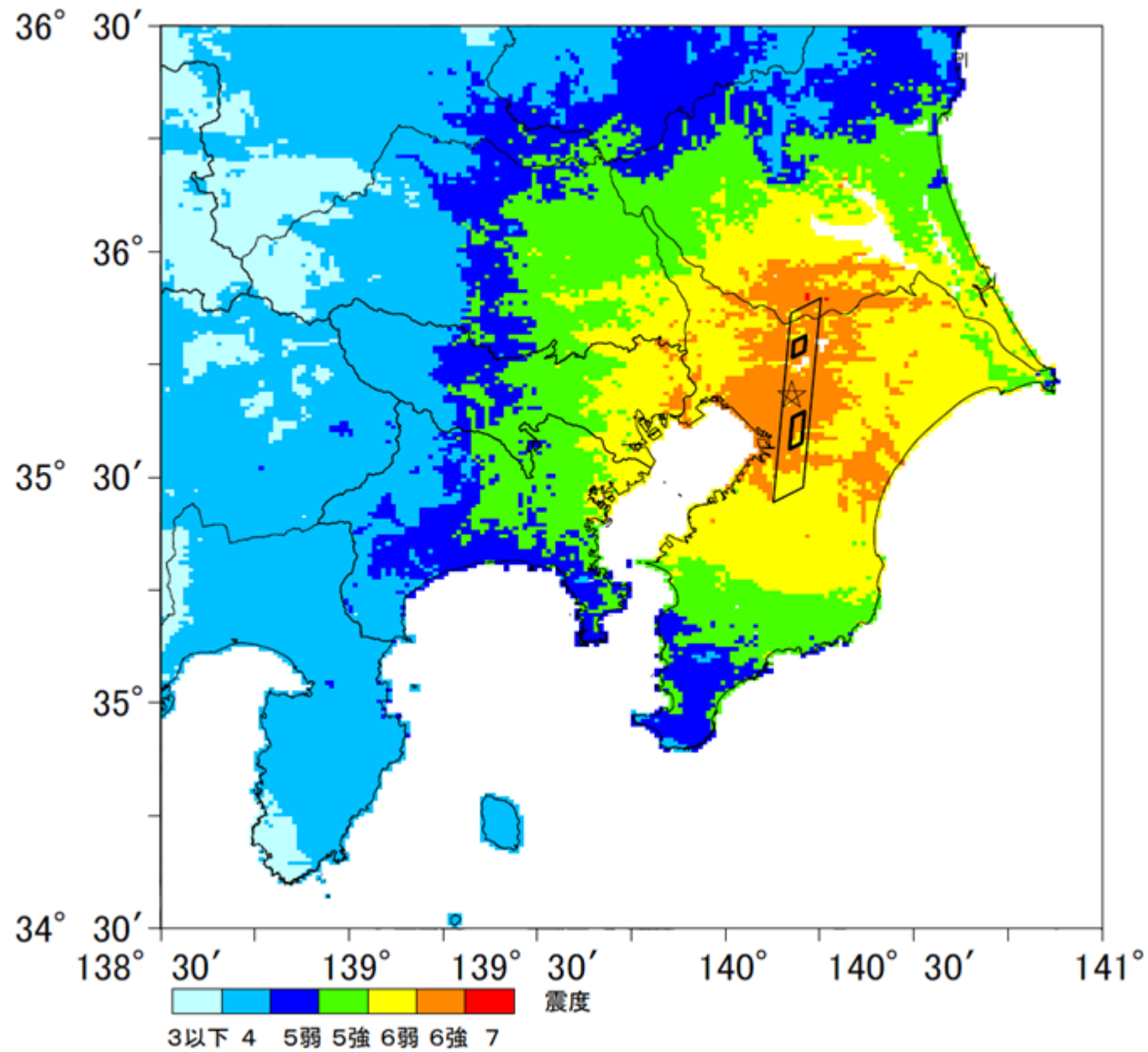
スラブ内地震の震度分布。(★は破壊開始点。)
