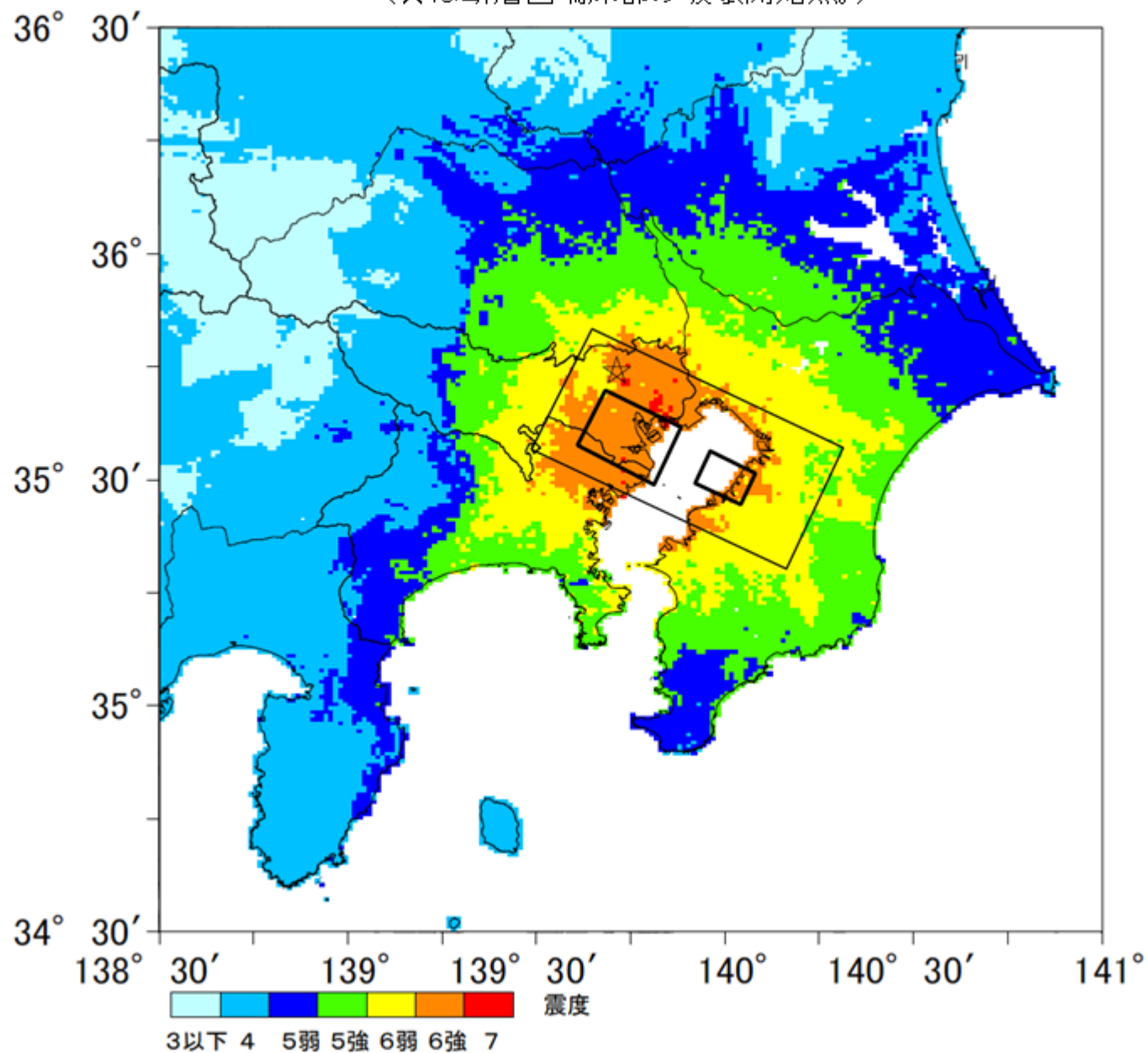
ケース3 浅いプレート境界を反映した東京湾北部地震の震度分布。 (★は断層西端深部の破壊開始点。)
