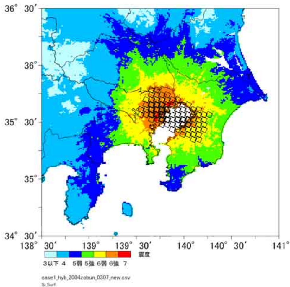
首都直下PJケース1の震度分布図
