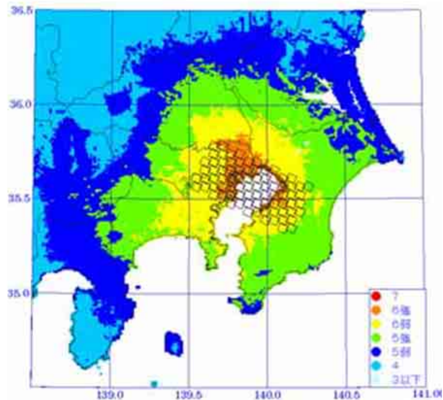
中央防災会議の震度分布図
