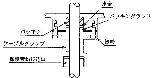
耐圧パッキン式引込方式
