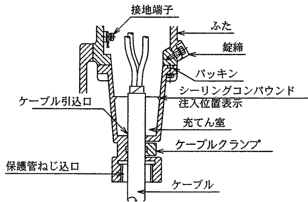
耐圧固着式引込方式
