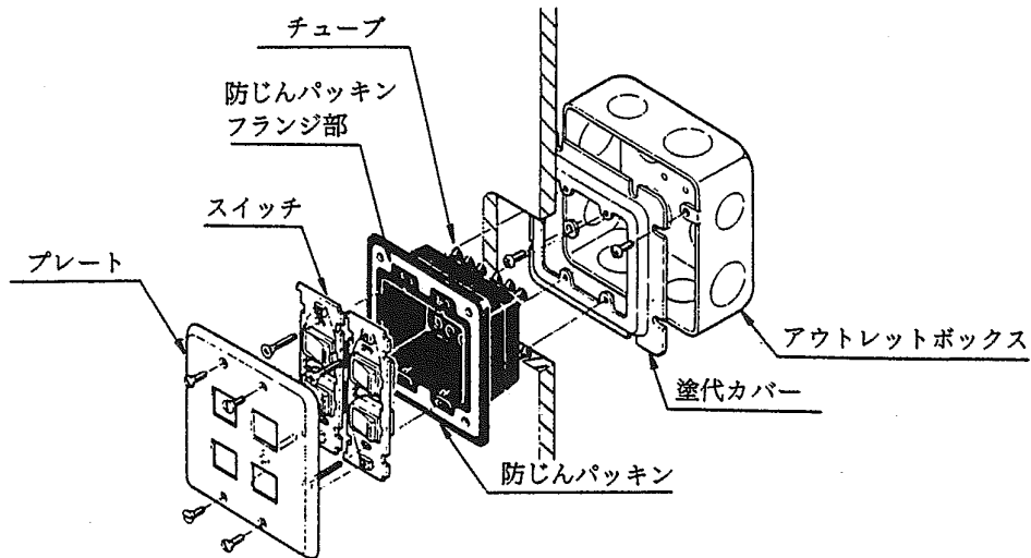
スイッチ取付け図
