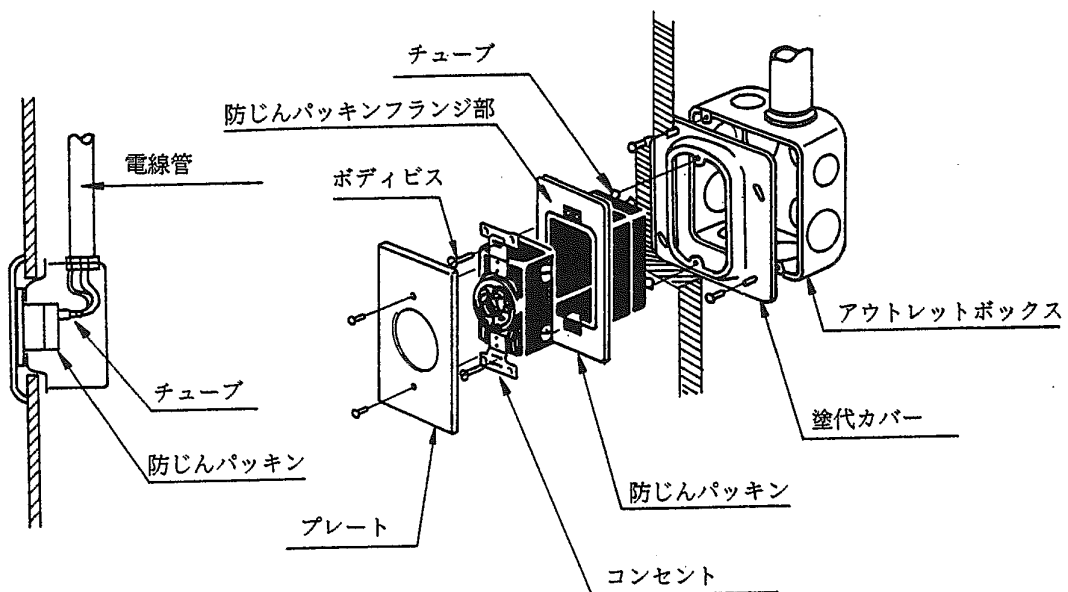
コンセント取付け図
