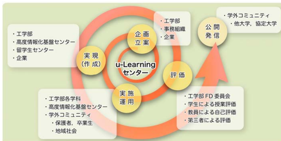
図4：組織構成
