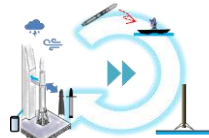
©JAXA
